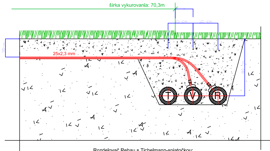
Rozdelovač Rehau s Tichelmann-spiatočkou: izolované PEHD potrubie d160/250
