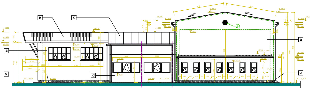
POHLAD SEVERNÝ M 1:100 - NAVRHOVANÝ STAV:
